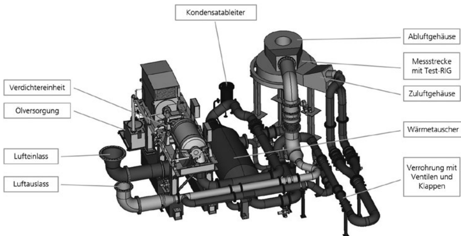
Bild 1.1 Beispielanlage – Darstellung ohne Schalldämpfer
