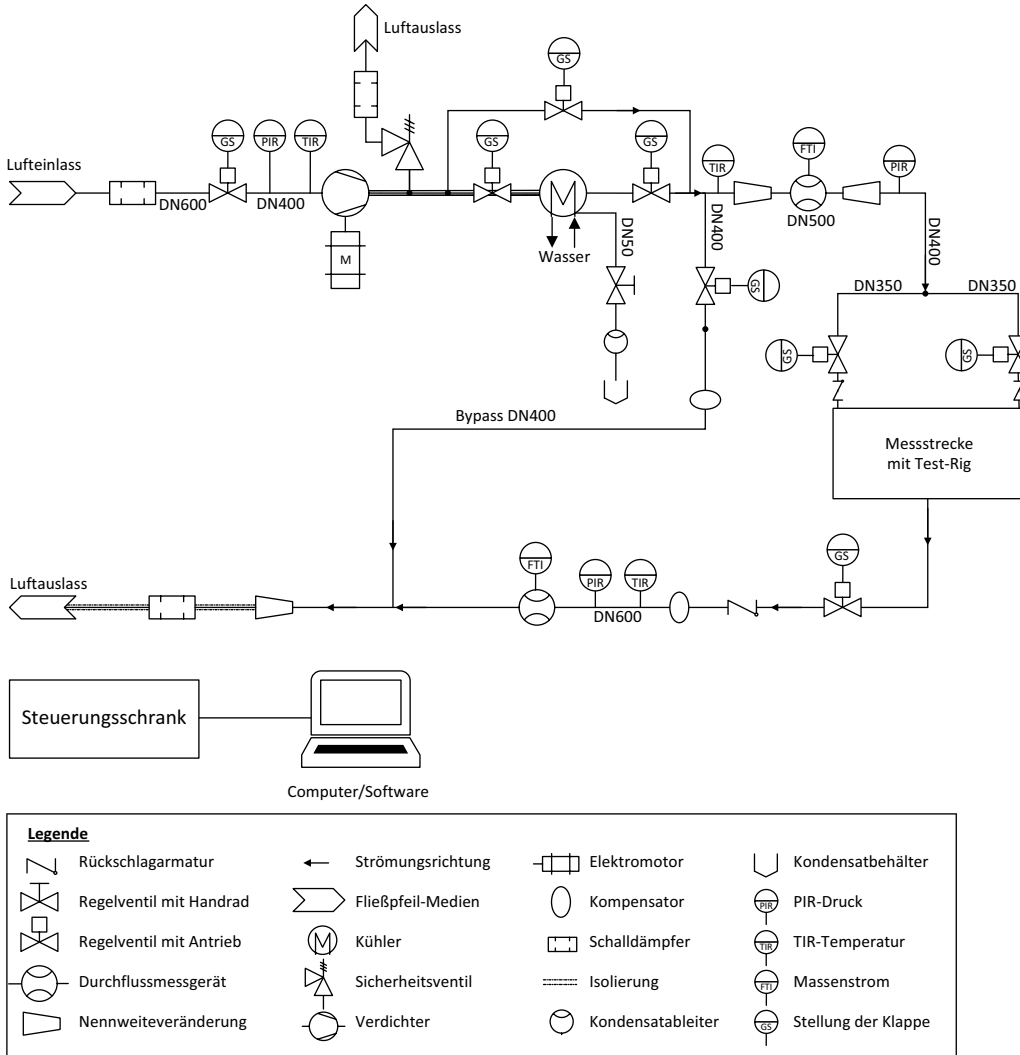
Bild 1.2 R&amp;I-Beispielanlage
