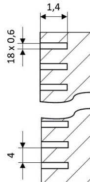
Abbildung 2: Abmessungen der im CAD generierten Schlitze
