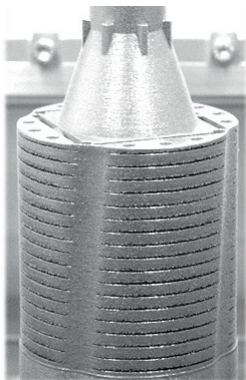
Abbildung 1: Additiv gefertigter Rotor einer PMSM aus FeSi3 mit integrierten umlaufenden Oberflächenschlitzen [17]
