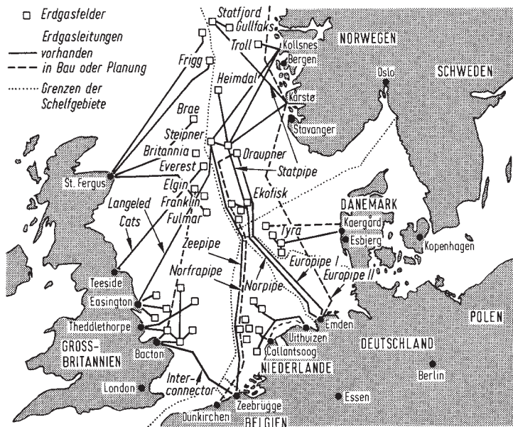
Bild 1.14 Erdgasfelder in der Nordsee (E.ON (a))
