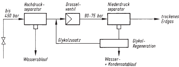
Bild 1.17 Prinzip einer Gastrocknung mit Glykol (gwf 1970)
