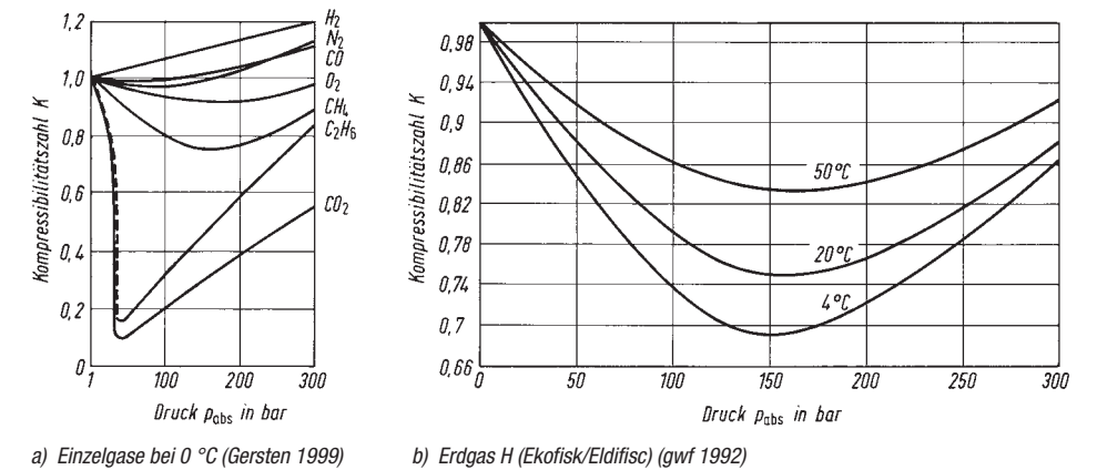
Bild 2.1 Kompressibilitätszahl K von Gasen
