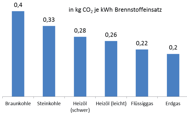
Bild 1.6 \text{CO}_2 -Abgabe bei der Verbrennung fossiler Energieträger: Heizwertbezogene Emissionsfaktoren 1 (E.ON (a))
