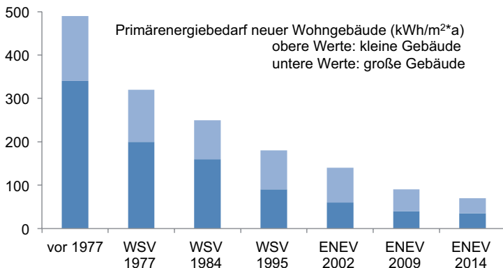
Bild 1.7 Entwicklung des zulässigen Primärenergiebedarfs von neuen Wohngebäuden (VDZ 2014)
