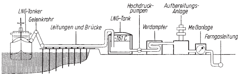
Bild 1.23 LNG-Anlandeterminal
