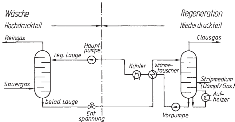
Bild 1.18 Entschwefelung von Saugergasen durch Gaswäsche nach dem Sulfinol-Verfahren (gwf 1982)
