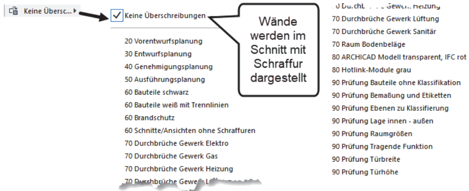
Abb. 1.14: Überschreibungsregeln
