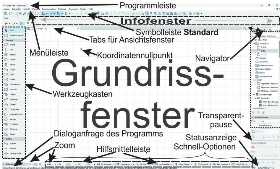
Abb. 1.6: Archicad-27-Bildschirm
