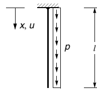
Bild 1.3 Einseitig festgehaltenen Dehnstab unter Eigengewicht
