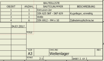
Abb. 1.6: Zeichnung der Explosionsansicht mit Positionsnummern und Stückliste
